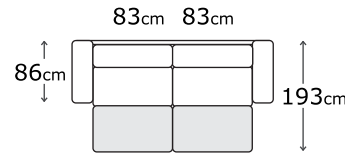
VUODESOHVA 3-OS
